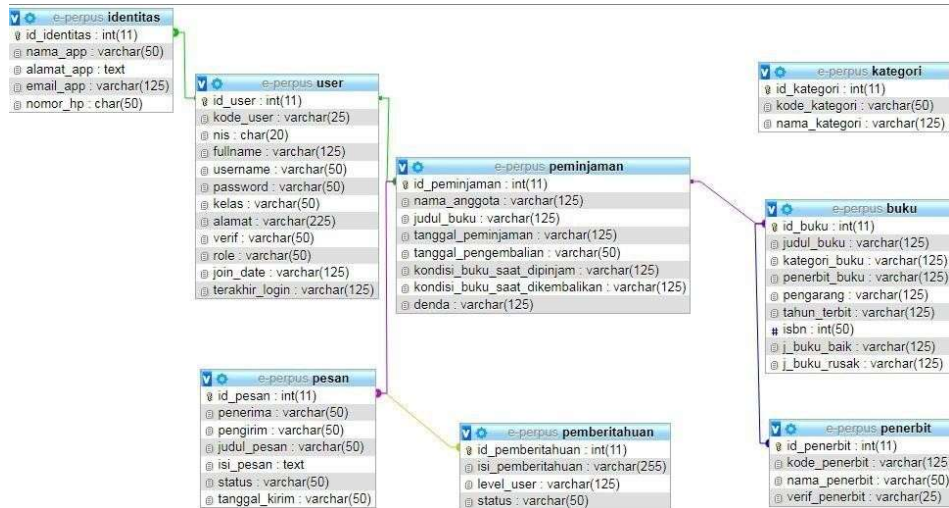
Gambar 3.6 Relasi Tabel
